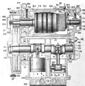
Fig. 2515. Top View.
